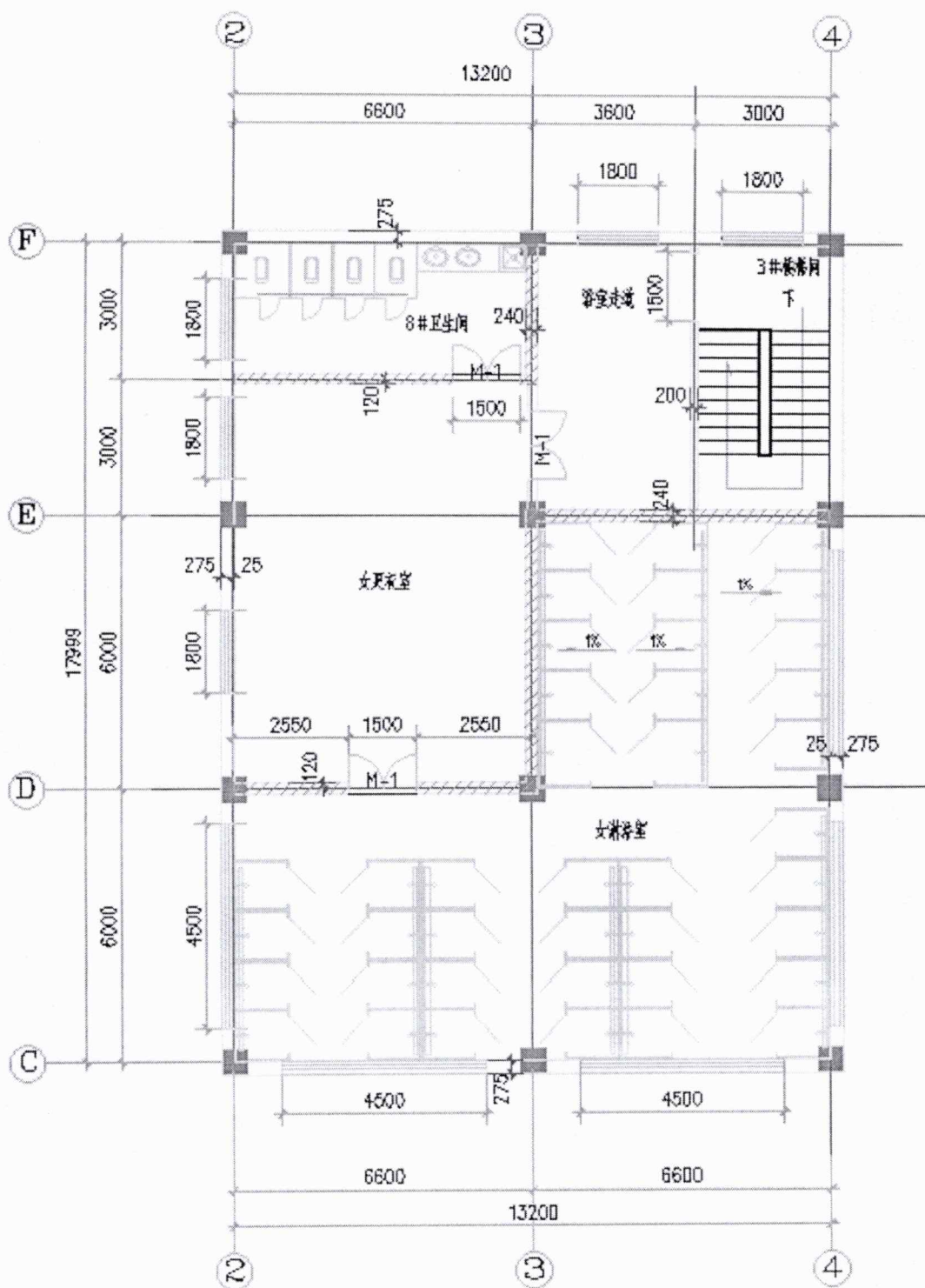
浴室二楼平面图
